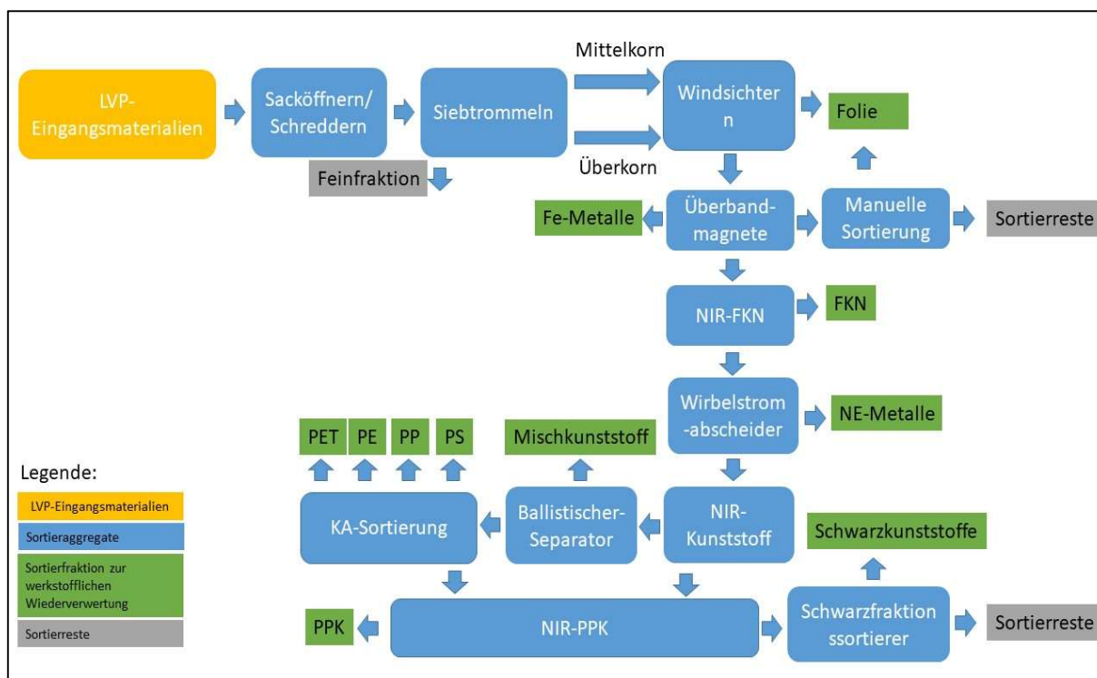
Abbildung 1 Allgemeines Verfahrensfliießdiagramm einer LVP-Sortieranlage, eigene Darstellung
